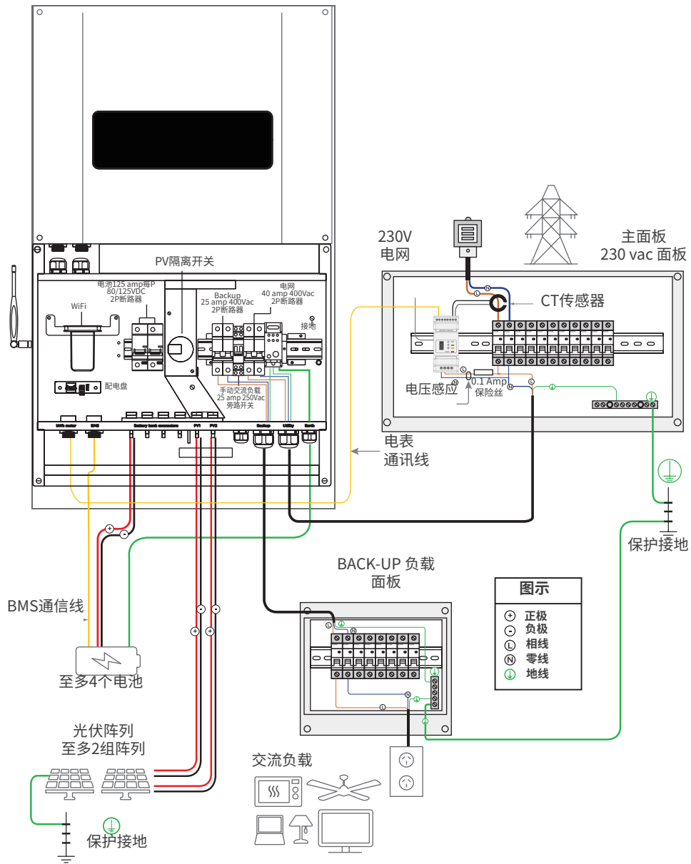
图11:接线系统
