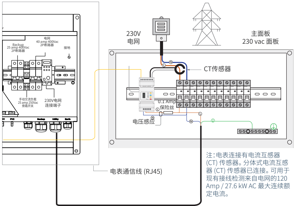
图20:电表接线
