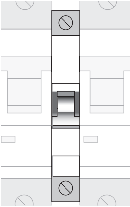
图 21: BACK-UP (I)位置的旁路开关
