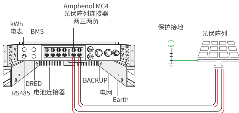
底部视图
