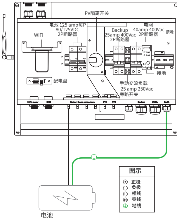
图14: 电池接线
