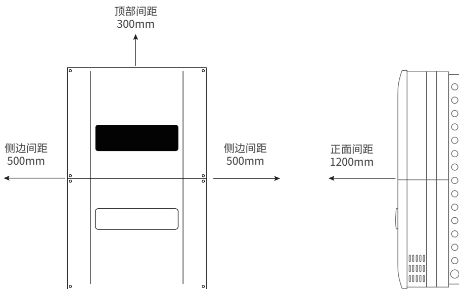
图二:最小间距要求
