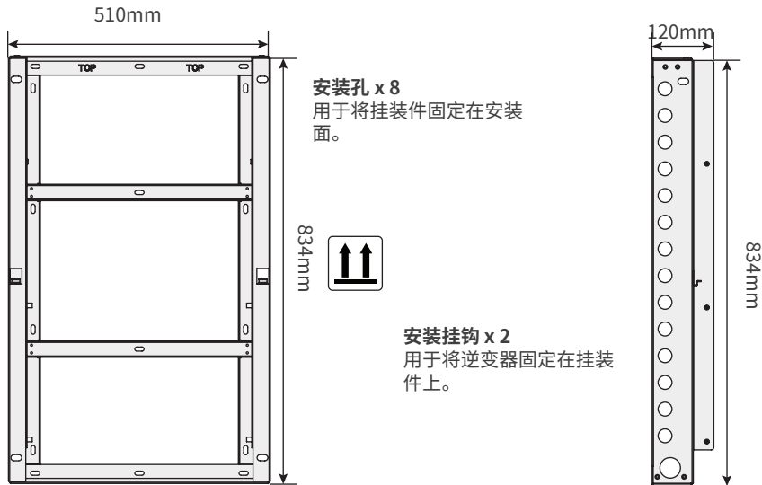
图5: 挂装件
