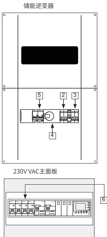
图25:关闭系统
