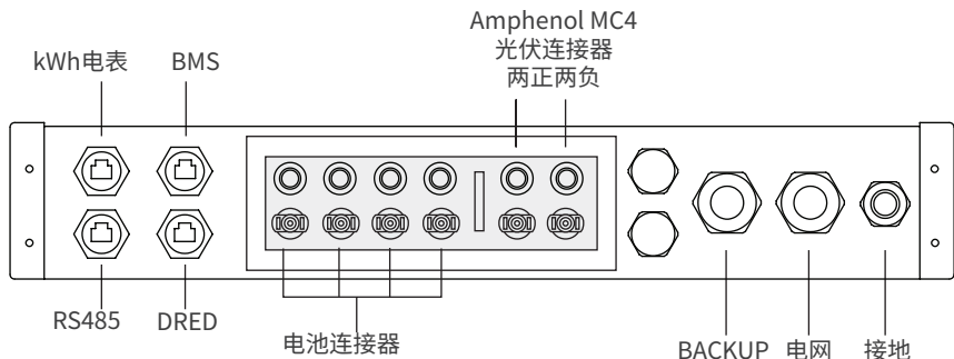
底部视图
