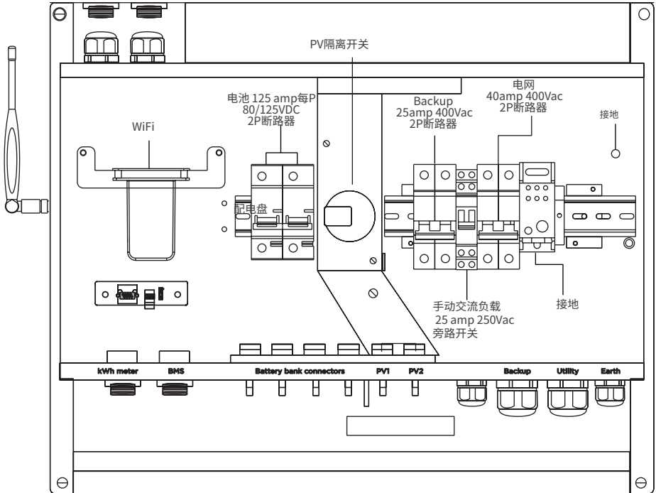
图16: 交流端子
