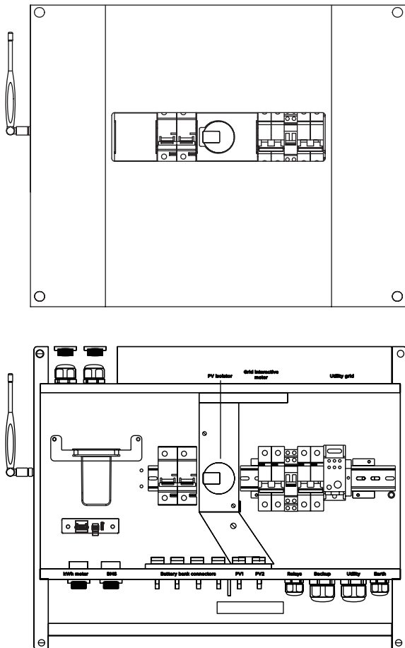
图9: 打开盖子
