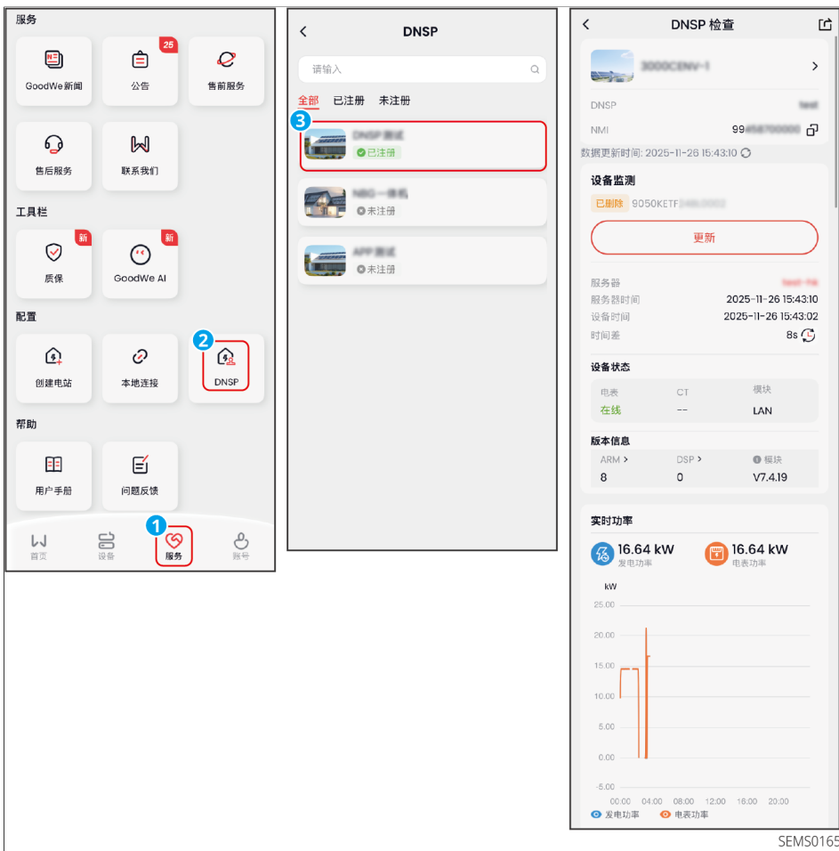
图37 DNSP校验
