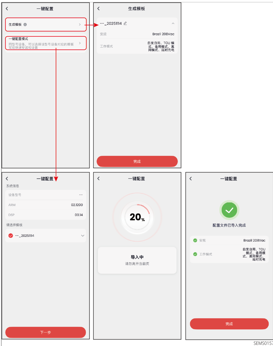
图25 一键配置
