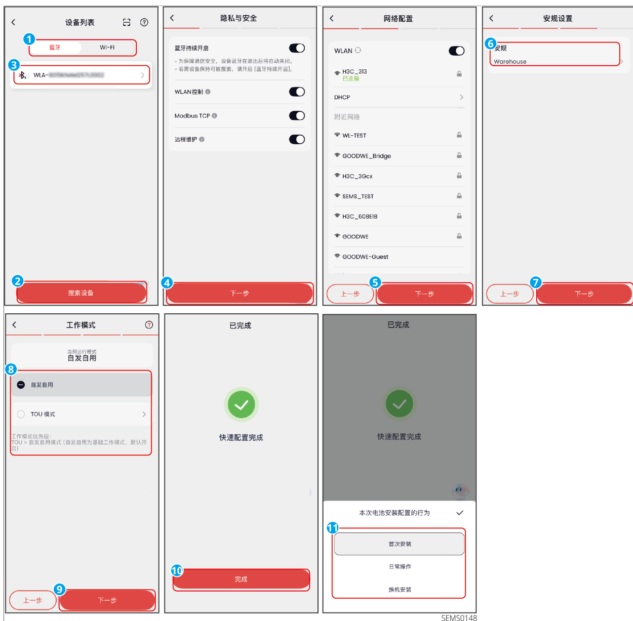
图6 快速配置设备
