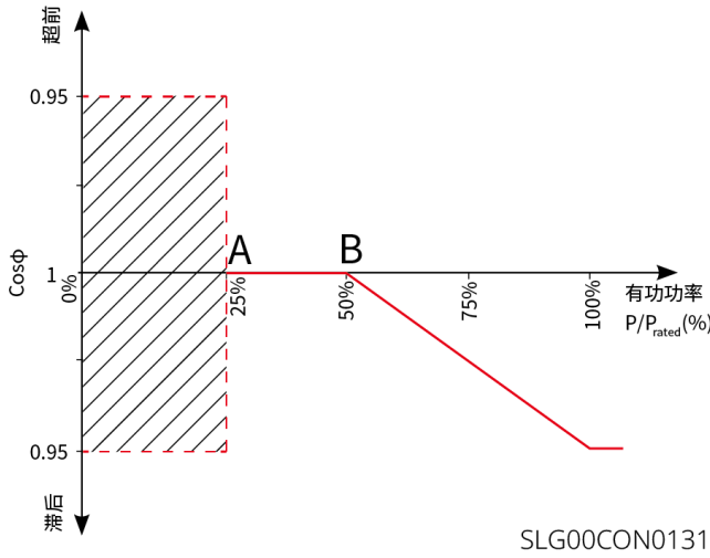
Cosφ曲线
