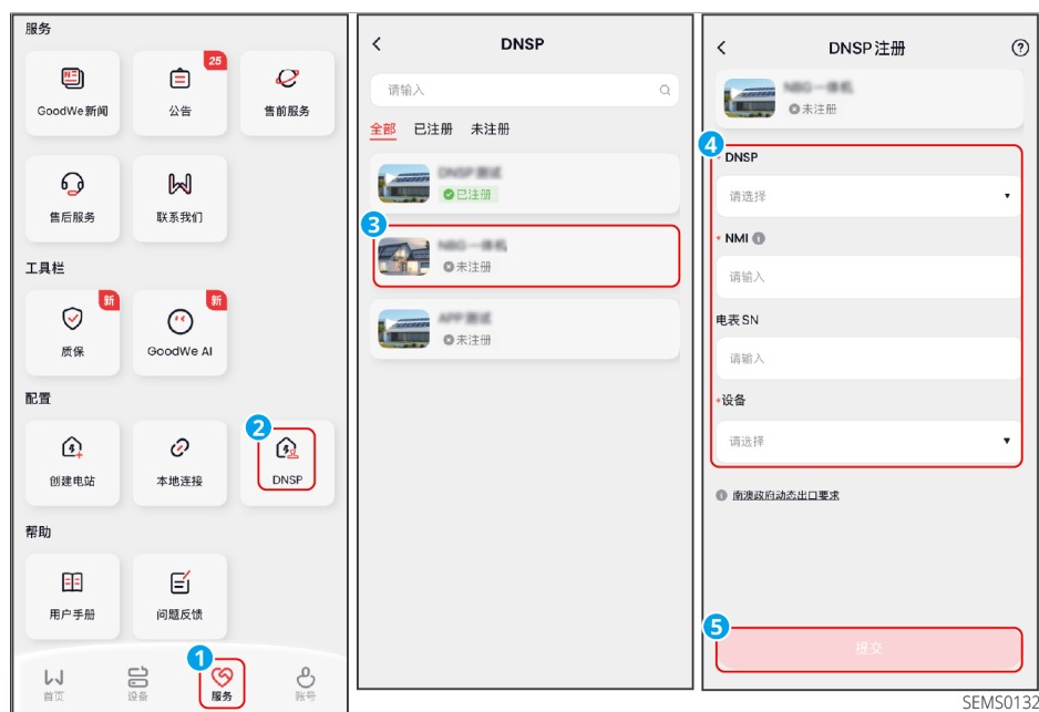
图36 DNSP注册
